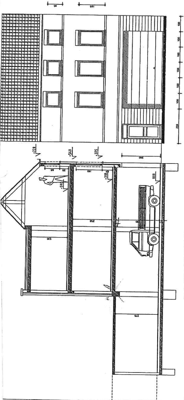
DOORSNEDE
